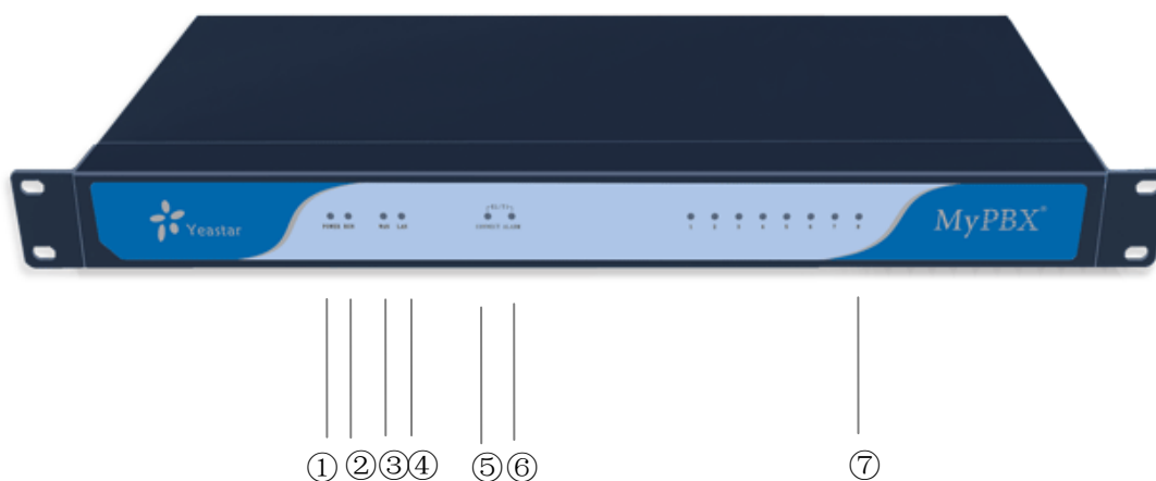
图1-2 MyPBX 前面板示意图
